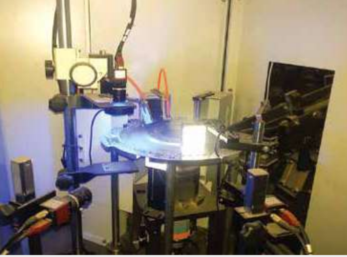
KAMERA SİSTEMLİ AYIKLAMA MAKİNASI
